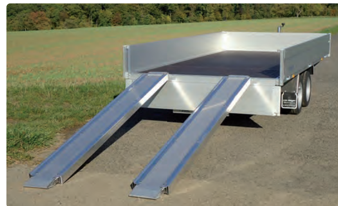
HLC 2741/186 Zubehör: Auffahrschienen, Klappkurbelstützen HLC 2741/186 Options : rampes, béquilles arrière (à relever) HLC 2741/186 Optional extras: skids, prop stands (with crank)
