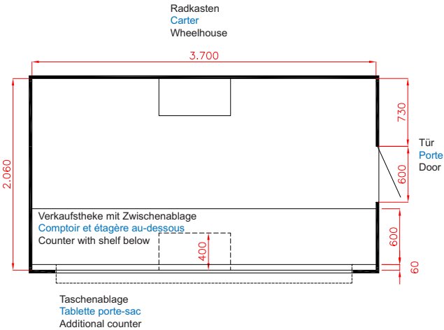
VKE 1337/206 Top Alle Maßangaben in Millimeter VKE 1337/206 Top Toutes les dimensions en millimètres VKE 1337/206 Top All measurements in millimetres
