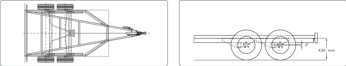
Chassis von oben: Anhänger spitz oder eckig, geschweißter, eingeschraubter V-Deichselrahmen (Stahl verzinkt), Aluprofile, Einstiegshöhe 430 mm Châssis vu d'en haut : panneau avant pointu ou plat, châssis en V (acier galvanisé) soudé et vissé aux profilés en aluminium, hauteur de chargement 430 mm Chassis from above: front panel V-shaped or flat, welded V chassis (galvanised steel), bolted to aluminium profiles, access height 430 mm
